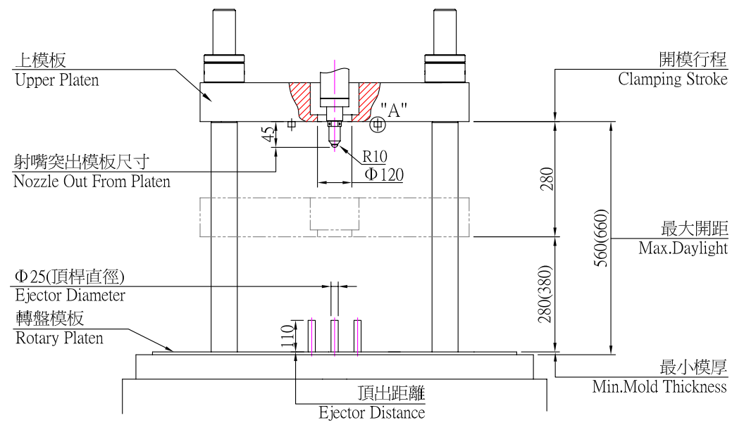
開合模規格示意圖(Clamping Unit Diagram)
