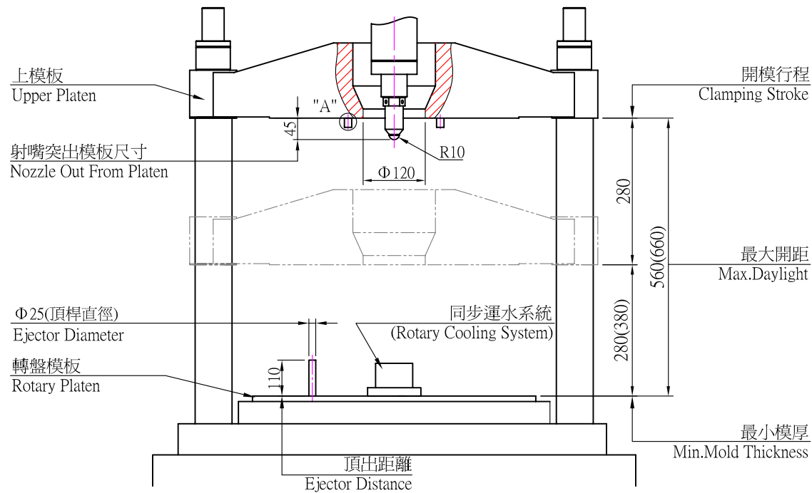
開合模規格示意圖(Clamping Unit Diagram)
