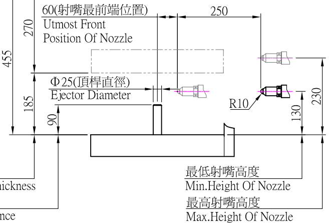
開合模規格示意圖(Clamping Unit Diagram)
