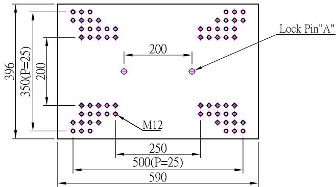
上模板(Upper Platen)
