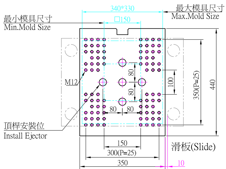
上模板(Upper Platen)
