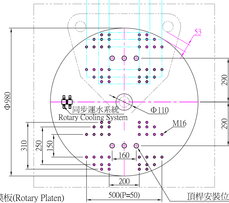
最小模具尺寸 Min.Mold Size
