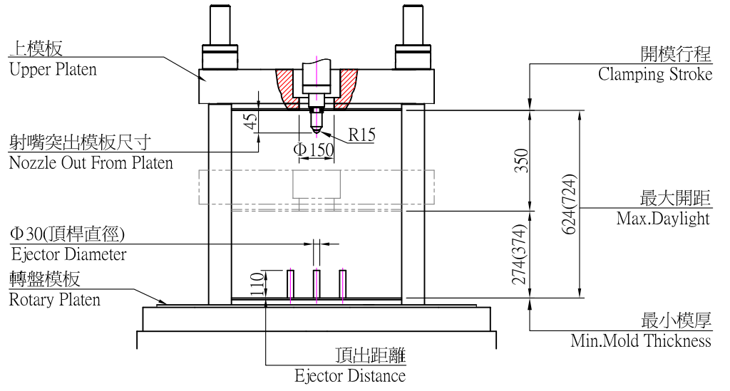
開合模規格示意圖(Clamping Unit Diagram)
