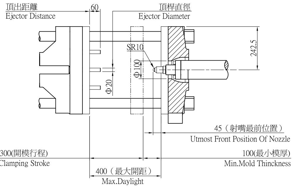
開合模規格圖示(Clamping Unit Diagram)
