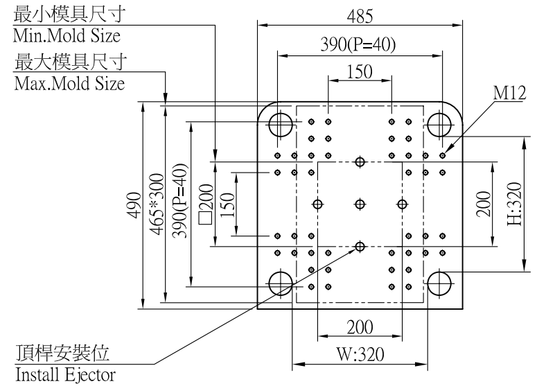
可動模板 (Movable Platen)
