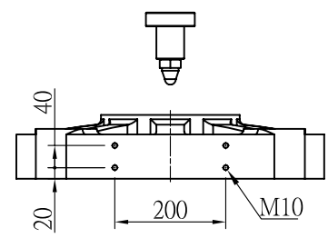
機械手安裝孔(Robot Mounting Holes)
