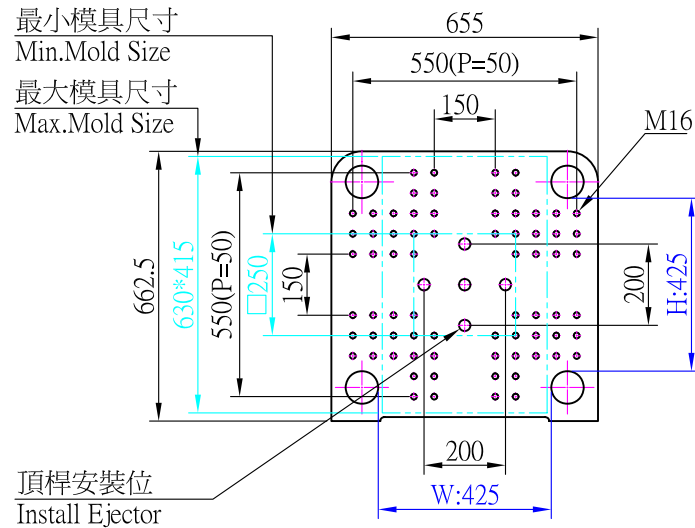
可動模板 (Movable Platen)
