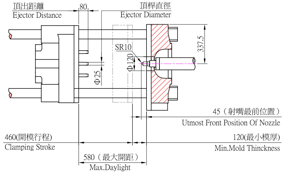
開合模規格圖示(Clamping Unit Diagram)
