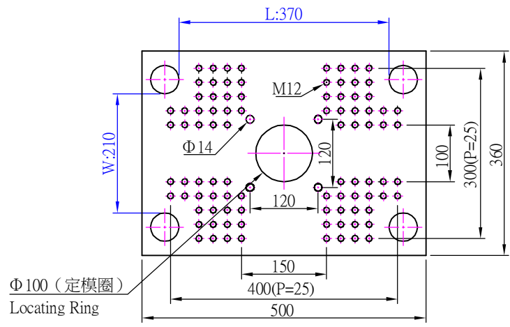
上模板(Upper Platen)
