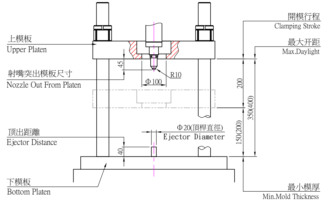
開合模規格示意圖(Clamping Unit Diagram)
