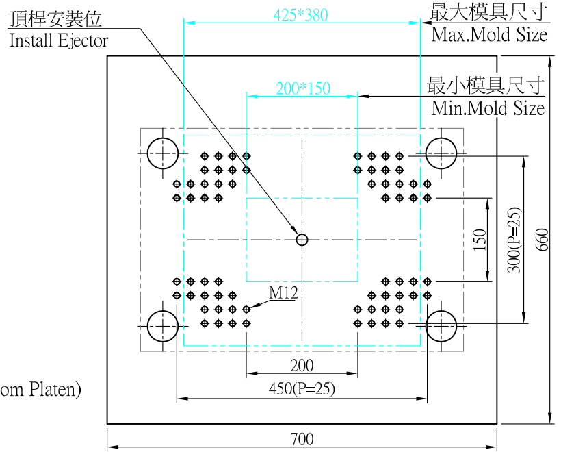
下模板(Bottom Platen)
